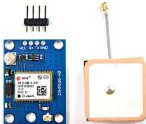
Fig. 3 GPS Module
