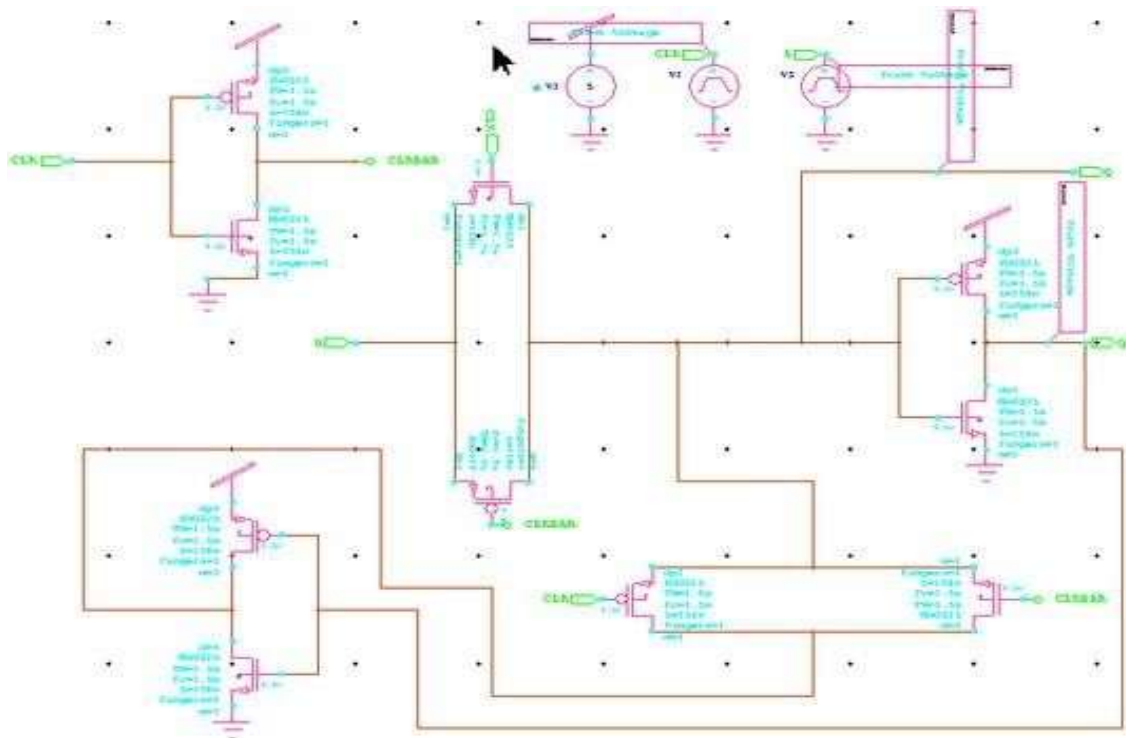
Fig4.3:D-FLIPFLOPUSINGTGSCHEMATIC
